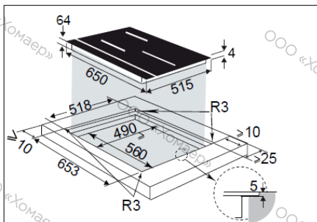
Монтаж заподлицо
