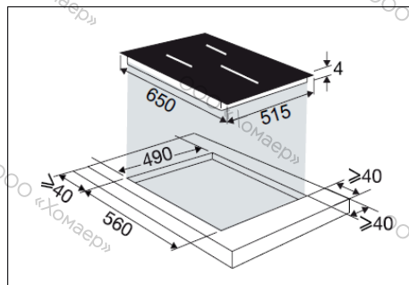
Накладной монтаж
